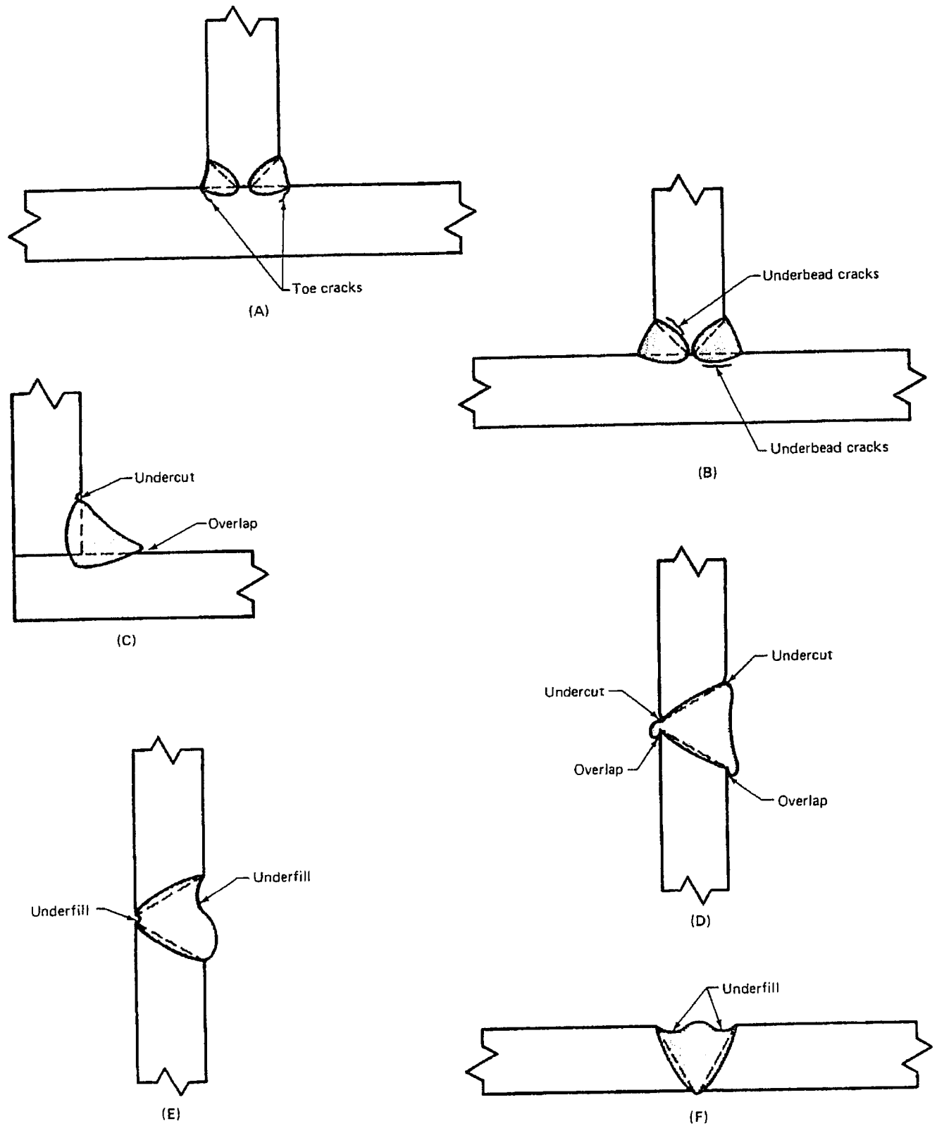
Fig. 24—Weld flaws
