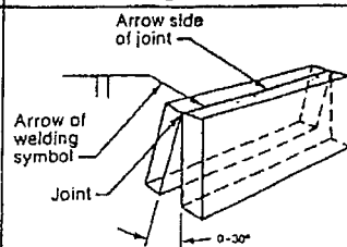
Edge Joint
