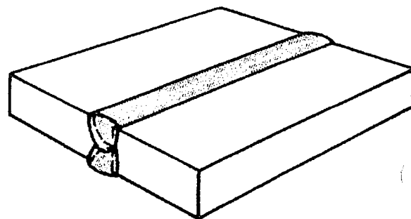
(D) Double-J-groove weld
