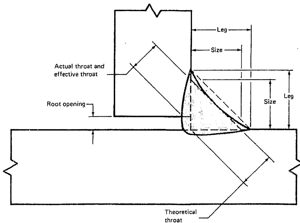
(D) T-joint with root opening
